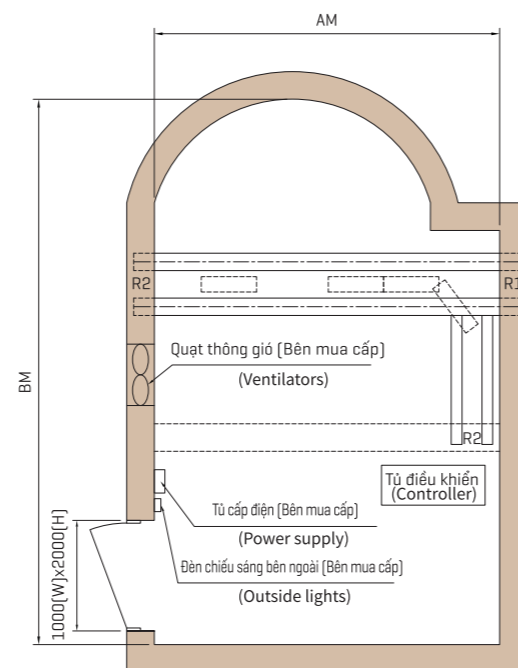
Mặt cắt ngang phòng máy (Machine room cross section)
