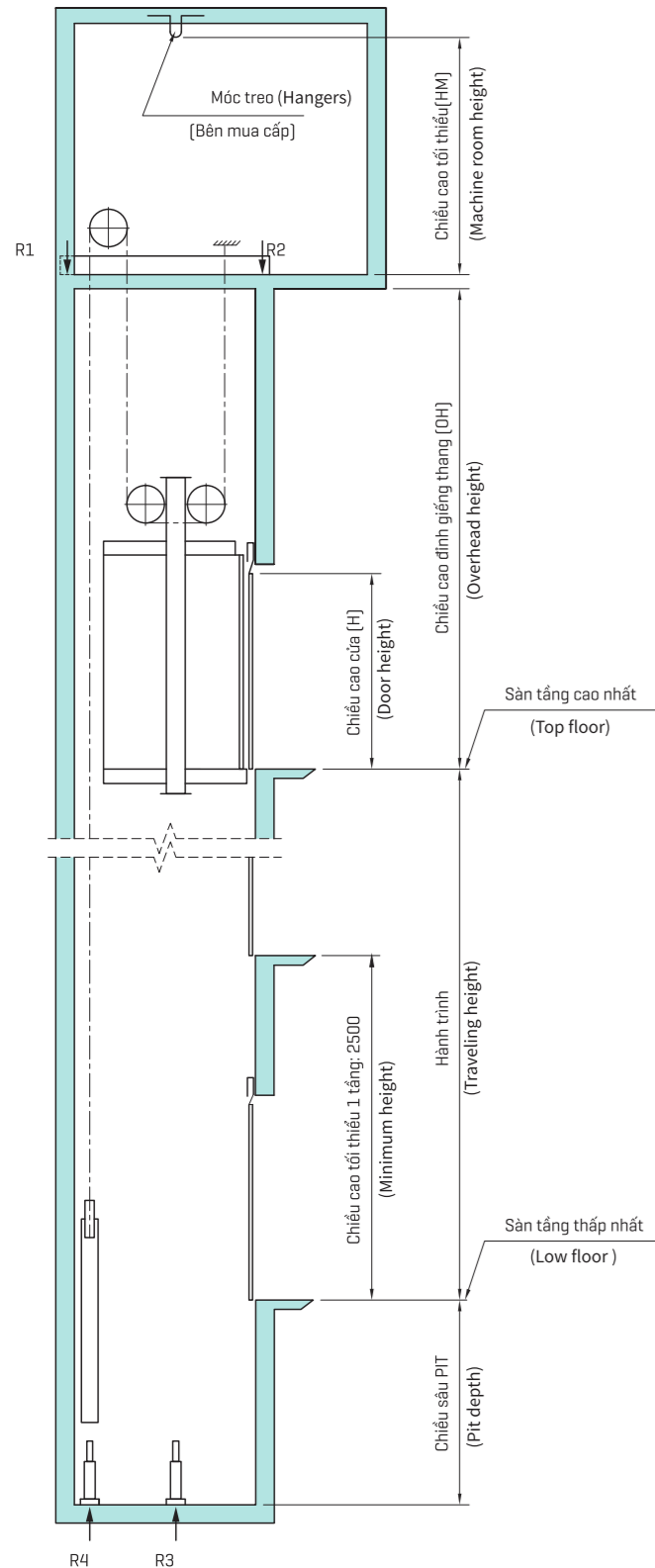
Mặt cắt đứng giếng thang (Hoistway sectional standing)
