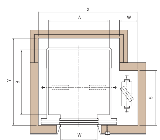
Mặt cắt ngang giếng thang hình vuông (Hoistway cross section)
